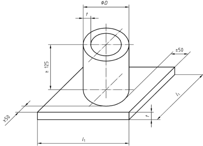
1.b: Boru köşe kaynakçısı sınav parçası minimum boyutları (Ölçüler mm'dir)
