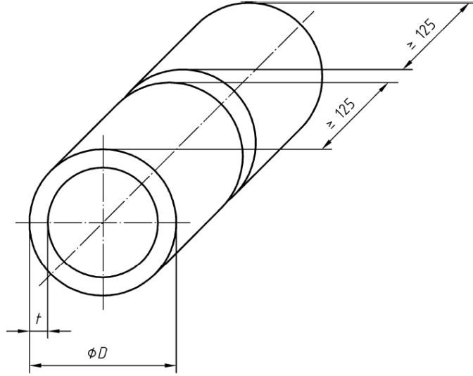
1.b: Boru köşe kaynakçısı sınav parçası minimum boyutları (Ölçüler mm'dir)
