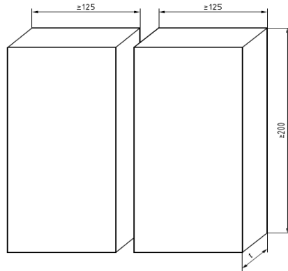
2.b: Plaka köşe kaynakçısı sınav parçası minimum boyutları (Ölçüler mm'dir)
